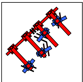
Bosquejo grada estrella, 2 hileras para Fendt GT 231 para cultivo de patatas u hortalizas. Construcción rígida especial del portaherramientas con soportes especiales para rejas descompactadoras, 4 estrellas por hilera.
